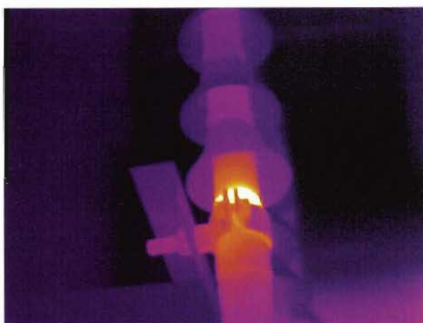
图 J. 28 35kV 交联电缆终端场强不均匀，发热
