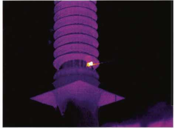
图 J.16 耦合电容器电容接头发热
