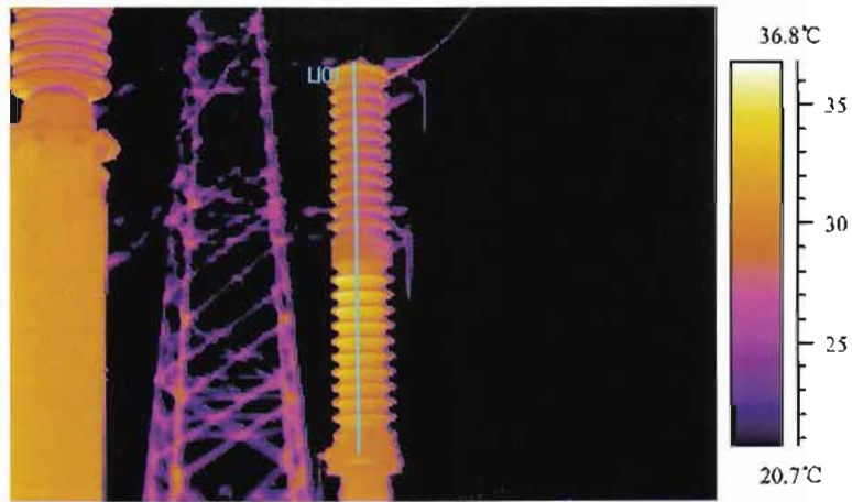
图 J.12 耦合电容器下节介质损耗偏大发热
