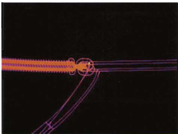
图 J. 41 500kV 线路线夹发热，接触不良
