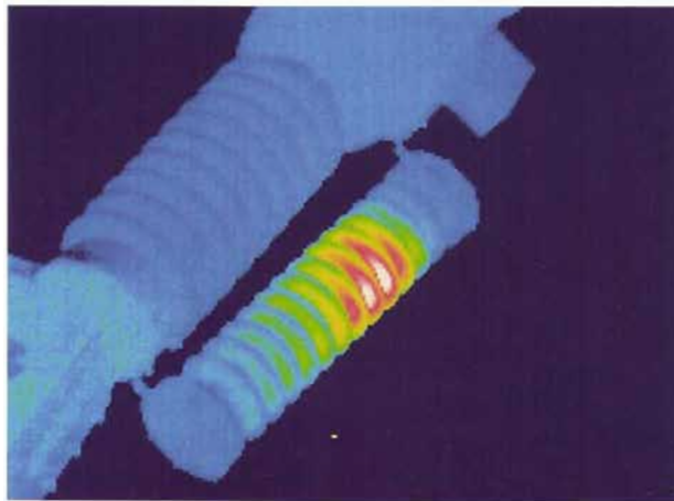
图 J.17 断路器并联电容发热
